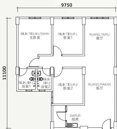
Pelan Lantai 平面图
